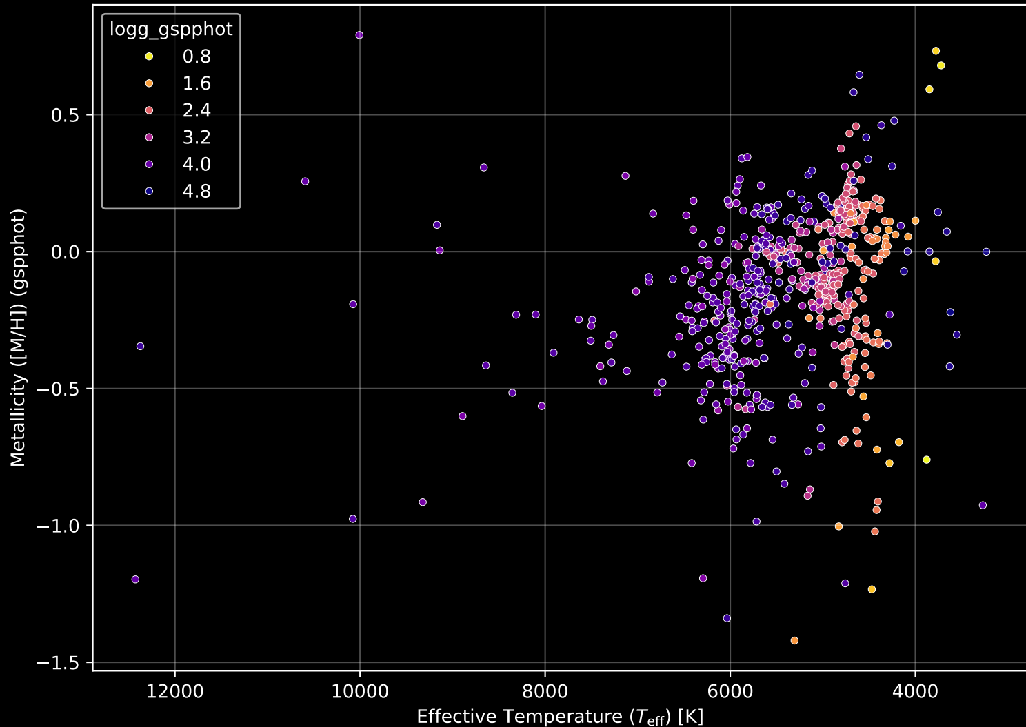
APOGEE DR17 Field: [K18_070+14] Stellar Population Parameters (n= 652)
